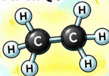
एथेन ( C_2H_6 )
